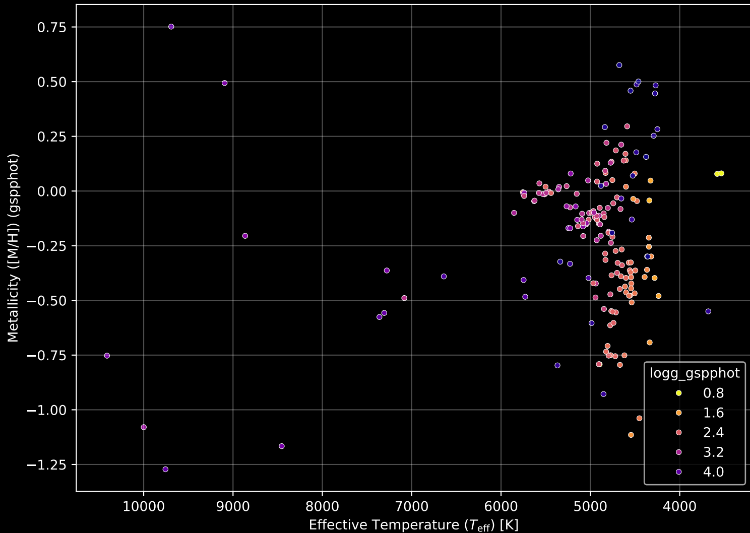
APOGEE DR17 Field: [N2204] Stellar Population Parameters (n= 175)
